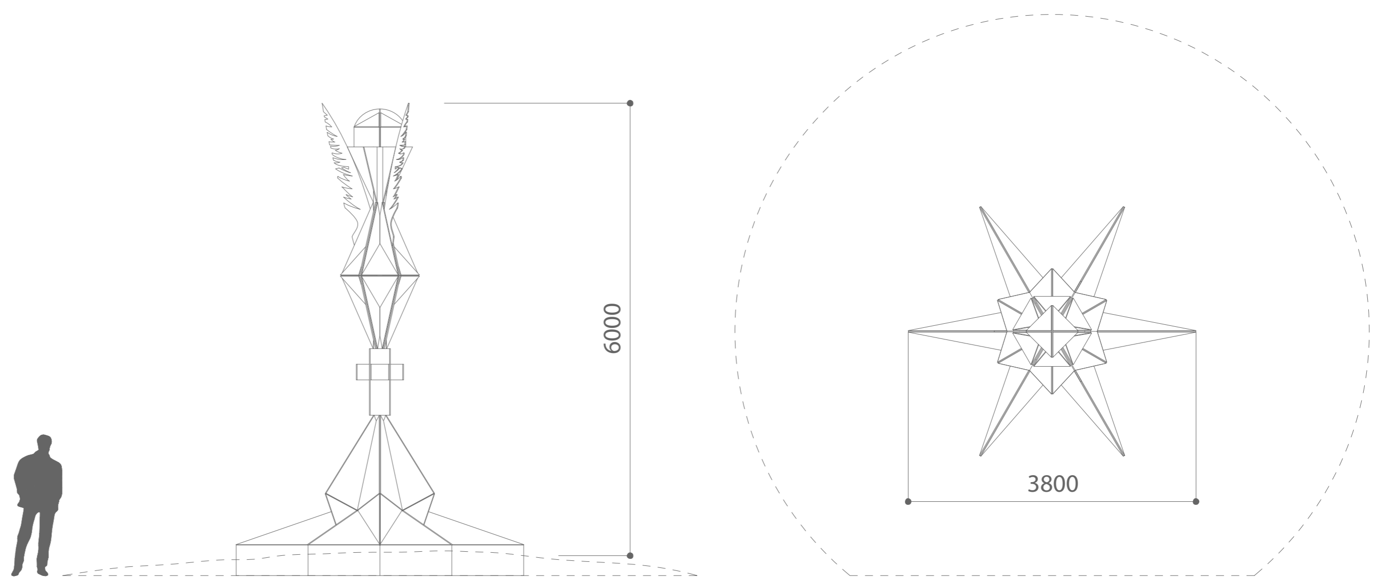
nárys, půdorys 1:50
